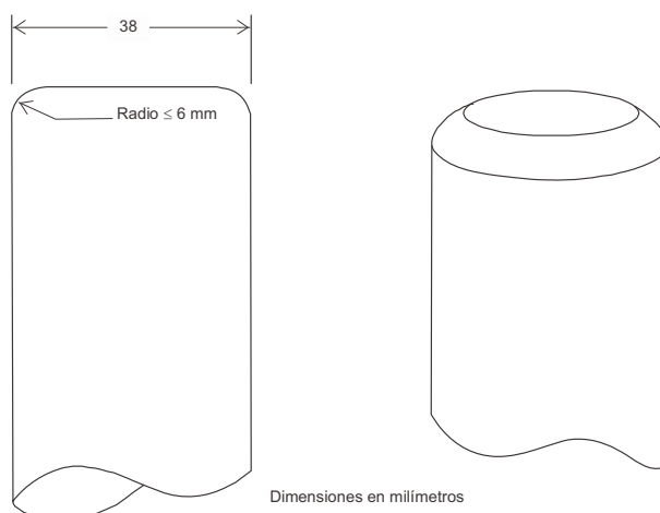
Figura 6-3. Vara de acero cilíndrica que se utiliza en el ensayo de penetración
