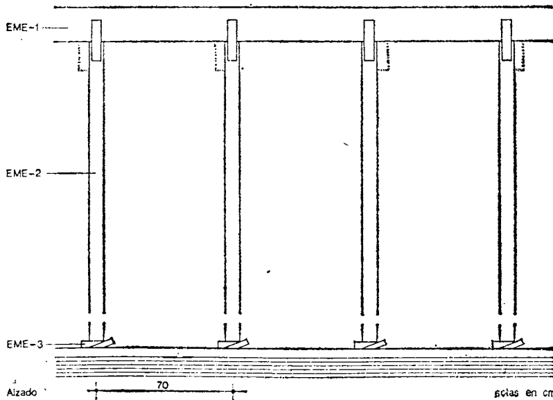
EME-3 Cuña.
