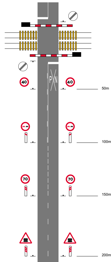
Figura 56 SEÑALIZACIÓN DE PASO A NIVEL CON BARRERA
