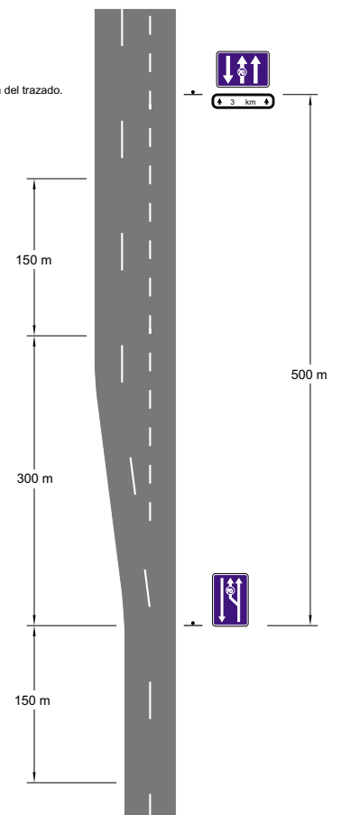
INICIO DE CARRIL ADICIONAL EN CARRETERA DE CALZADA ÚNICA
