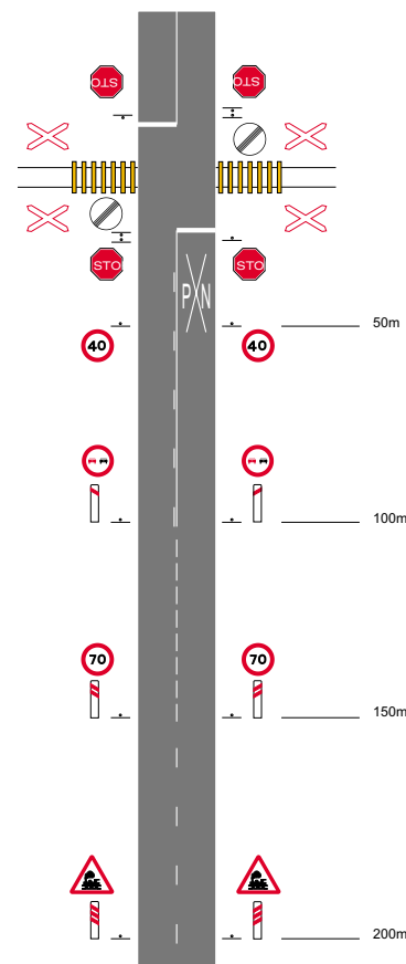
Figura 57 SEÑALIZACIÓN DE PASO A NIVEL SIN BARRERA
