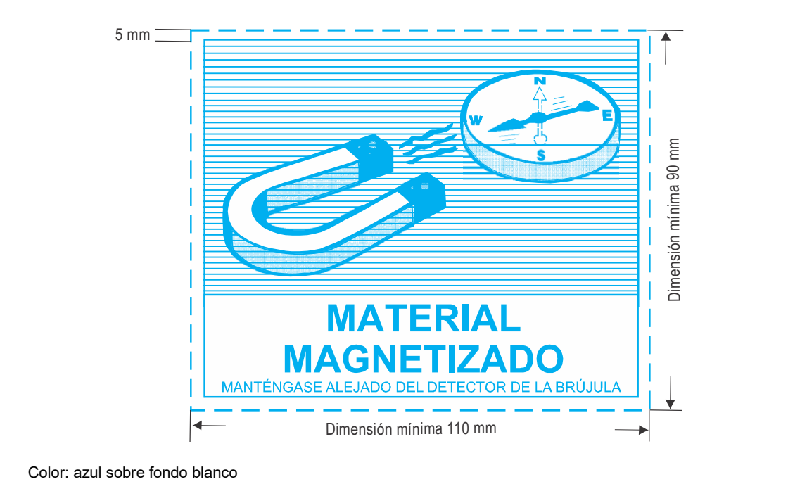
Figura 5-27. Material magnetizado
