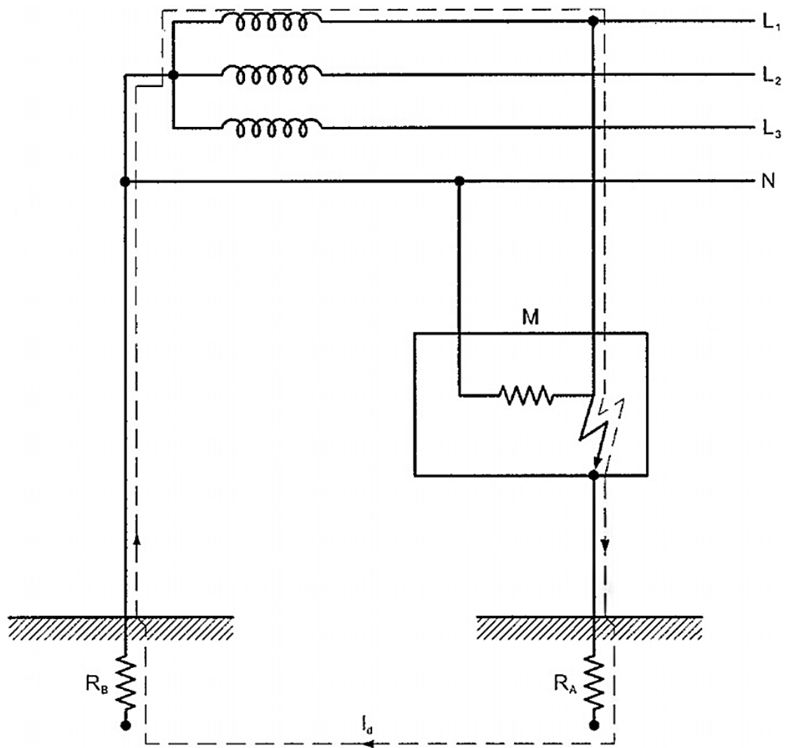
Figura 4. Esquema TT
