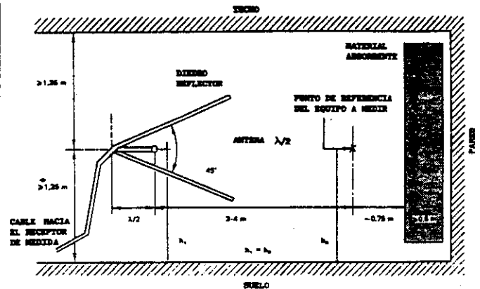
FIGURA 1. Sala de pruebas (representada para polarización horizontal).
