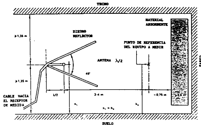
FIGURA 1. Sala de pruebas (representada para la polarización horizontal).
